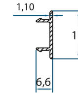
DİKME VİDA KAPAĞI SEWING SCREW COVER 2876 0.085 kg/m
